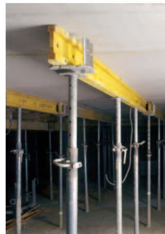
Bild 3 und 4: Montageunterstellung
