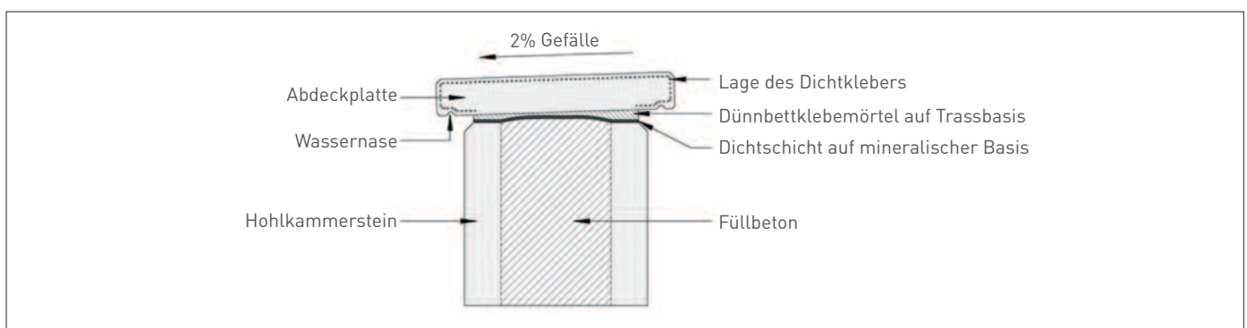
Abbildung 8: Skizze Dichtschicht und Abdeckplatte
